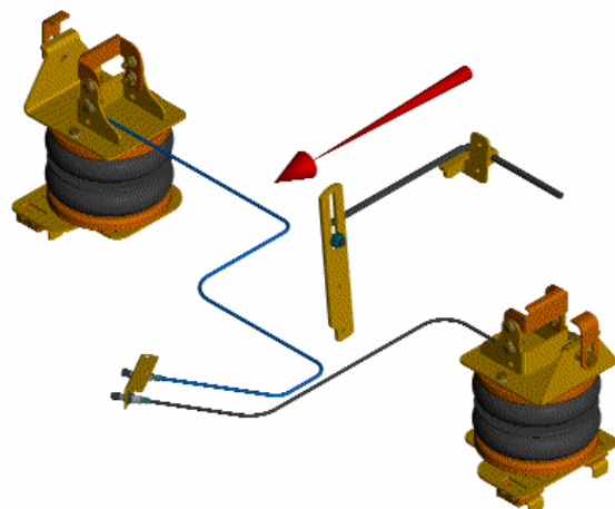
Schéma 1(c) Configuration pour véhicule équipé d'une butée caoutchouc abaissée
