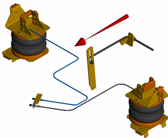
Schéma 1(b) Configuration pour véhicule équipé d'une butée caoutchouc standard
