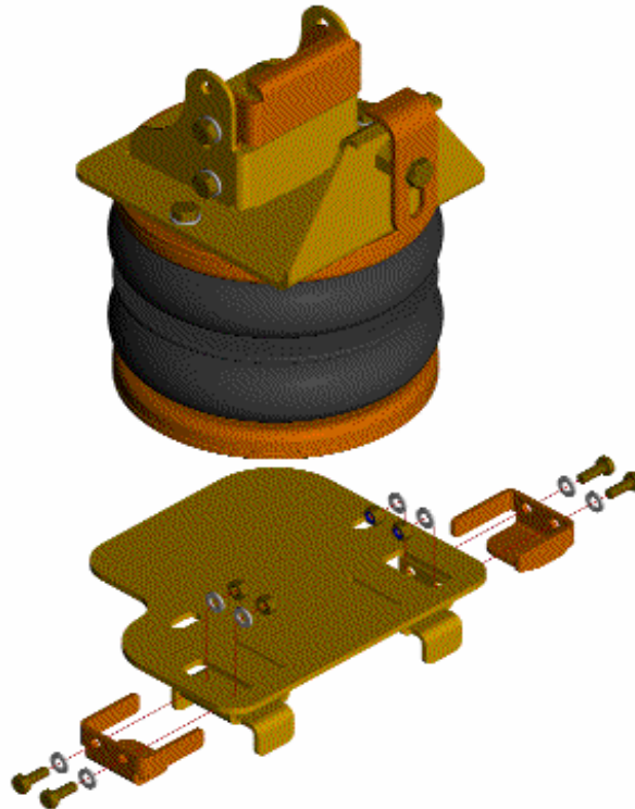
Schéma 1(a). Coussin et supports
